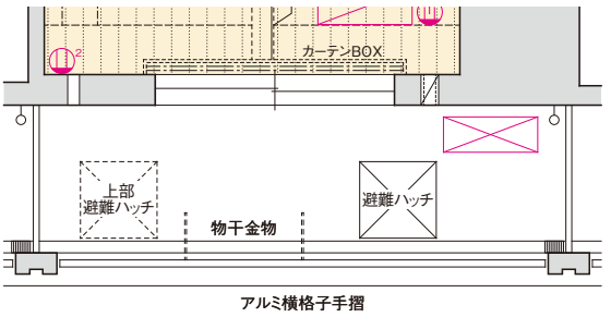
■Bタイプ(3階)部分図
